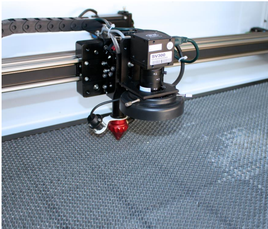
A kamera a lézerfej mellett. Az egyszeri szkennelési terület 100*100 mm / The camera is installed at the right side or front of the laser head. Its single scan area is 100x100mm.
