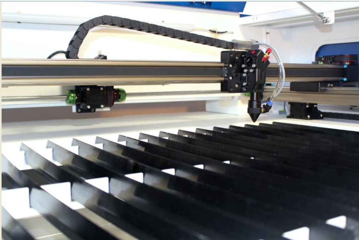
A kamera a lézerfej mellett. Az egyszeri szkennelési terület 100*100 mm / The camera is installed at the right side or front of the laser head. Its single scan area is 100x100mm.
