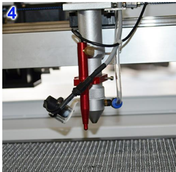
Vörösfényű jelölő és autó fókuszs a lézerfejnél / Red pointer and auto focusing (opció)
